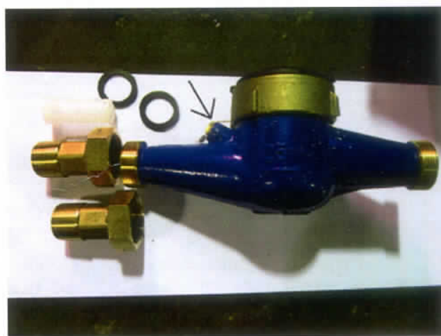
Рисунок 2 – Схема пломбировки от несанкционированного доступа, обозначение места нанесения знака поверки счетчиков холодной воды крыльчатых ВДХ-М, ВДХ-ИМ, турбинных ВДТХ-М, ВДТХ-ИМ, холодной и горячей воды крыльчатых ВДГ-М, ВДГ-ИМ, турбинных ВДТГ-М, ВДТГ-ИМ
