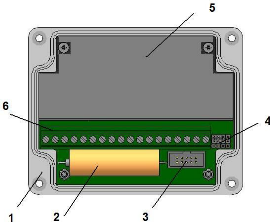
Рис.7. Конструкция тепловычислителя ВТЭ-2К.
