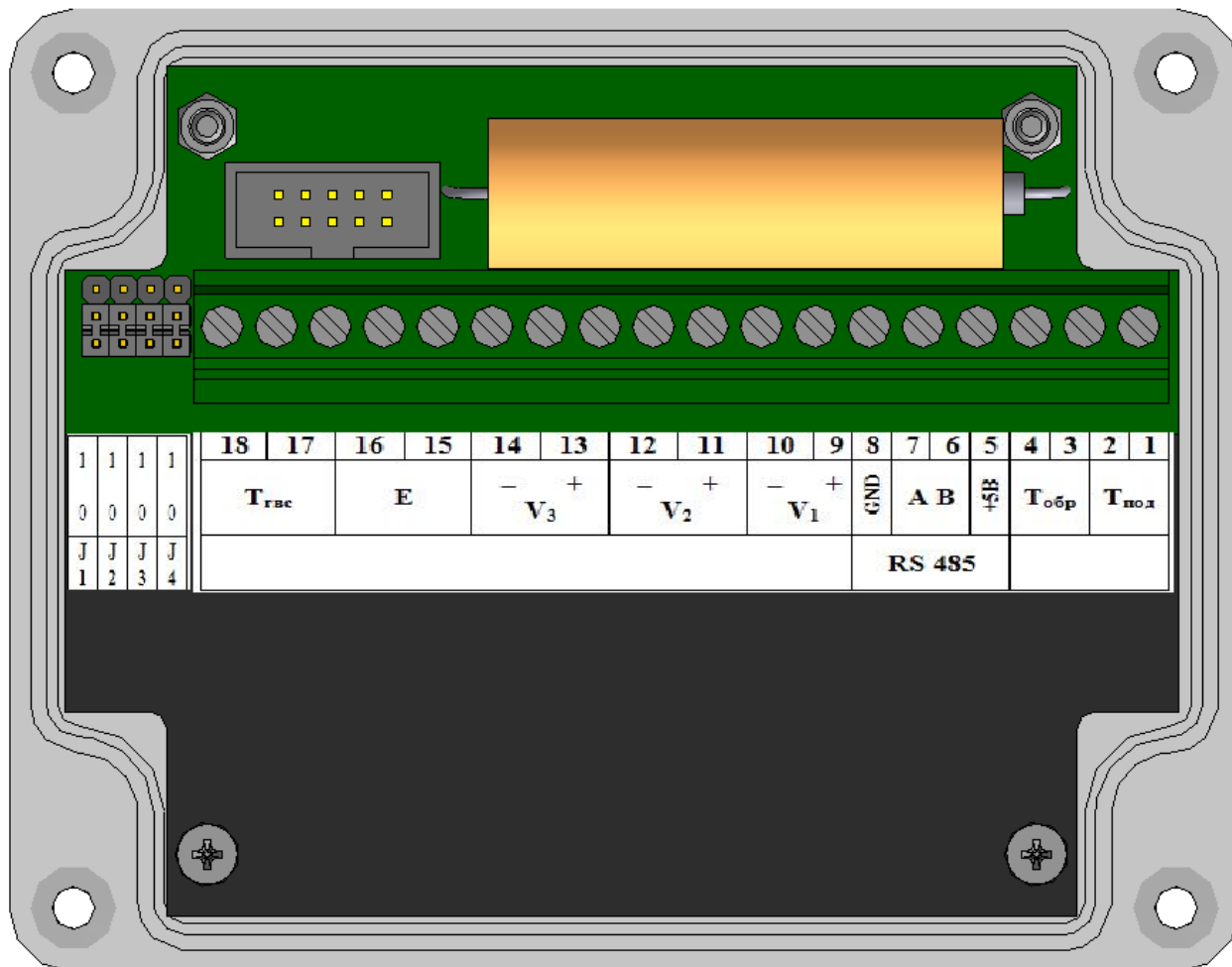
Рис.13 Расположение клемм ВТЭ-2 (модификация СТ 20 К)
