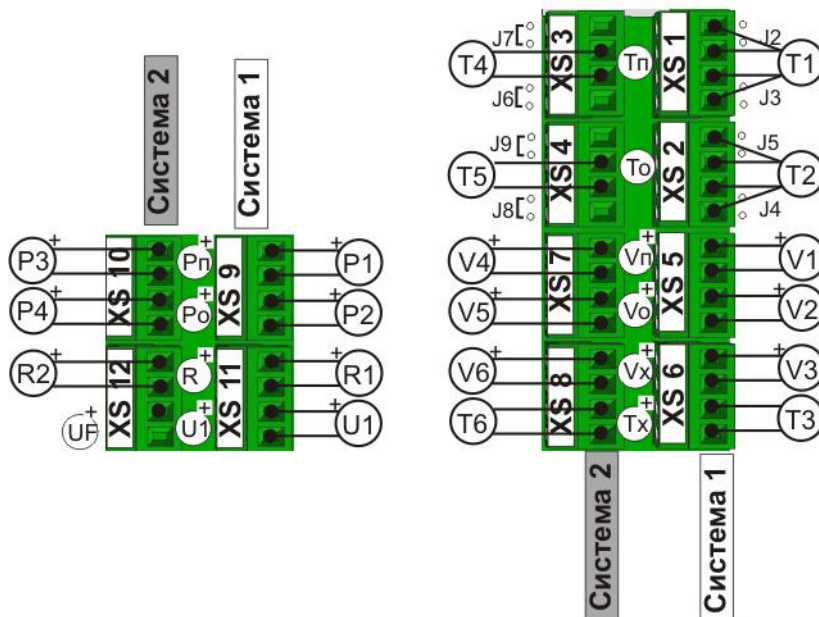
Рис.11. Схема подключения вычислителя ВТЭ-2 (модификация СТ 20 ПМ)
