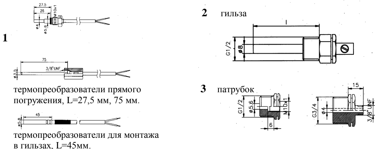
Рис.9. Варианты конструктивного исполнения термопреобразователей сопротивления Pt500 и крепежных элементов для них.
