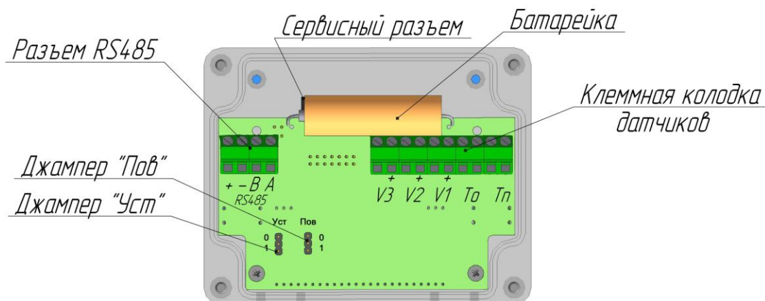
Рис.5. Конструкция тепловычислителя ВТЭ-2К-М.
