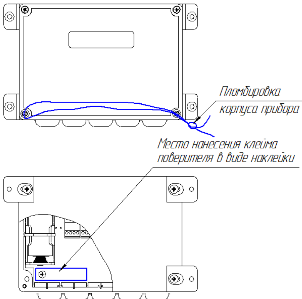
Рис. 8 Схема пломбировки корпуса и платы вычислителя
