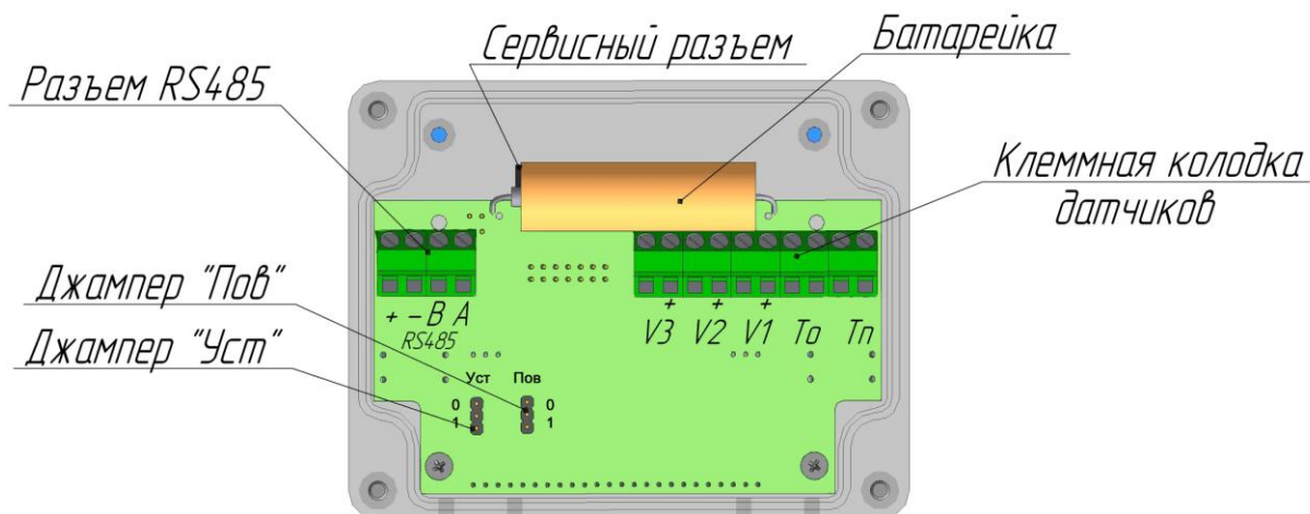
Рис.15. Расположение функциональных переключателей ВТЭ-2 (модификация СТ 20 К-М)
