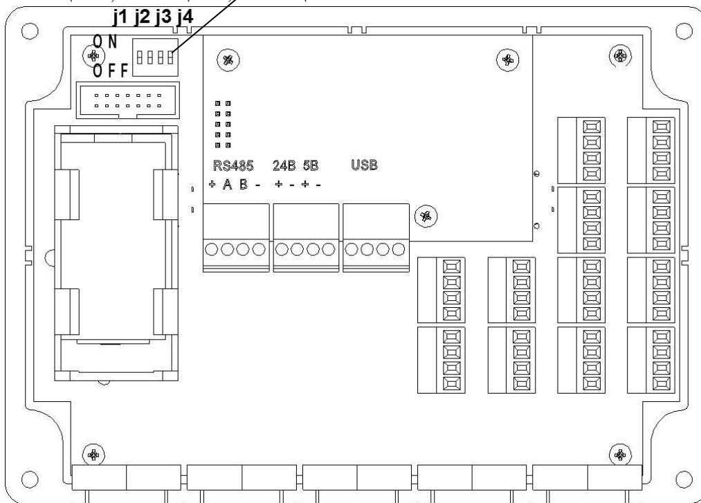
Рис.14. Расположение функциональных переключателей ВТЭ-2 (модификация СТ 20 ПМ)
