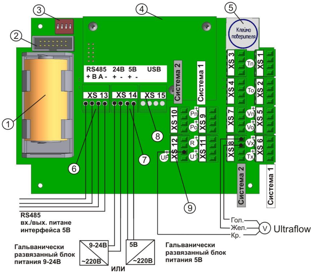
Схема подключения 2х проводная
