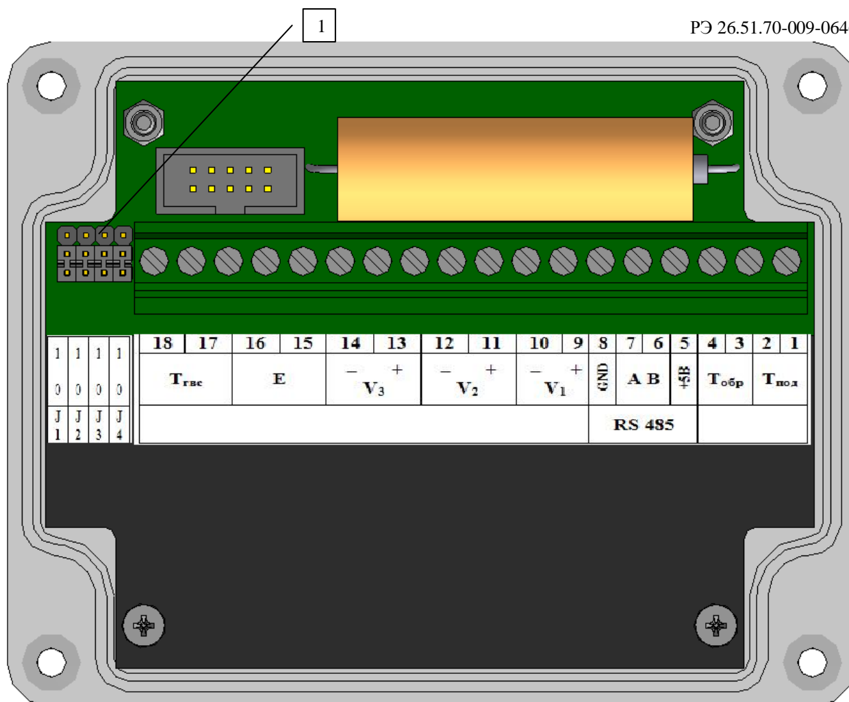
Рис.16. Расположение функциональных переключателей ВТЭ-2 (модификация СТ 20 К)
